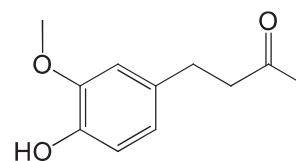
Zingerone
