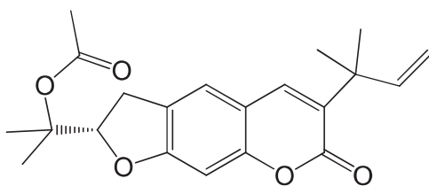
Rutamarin
