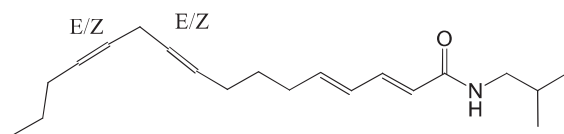
60
